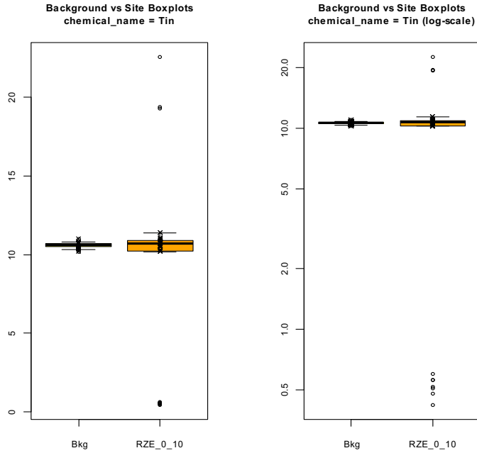
RZE – Background Data (0-10 fbg), Site Data (0-10 fbg)
